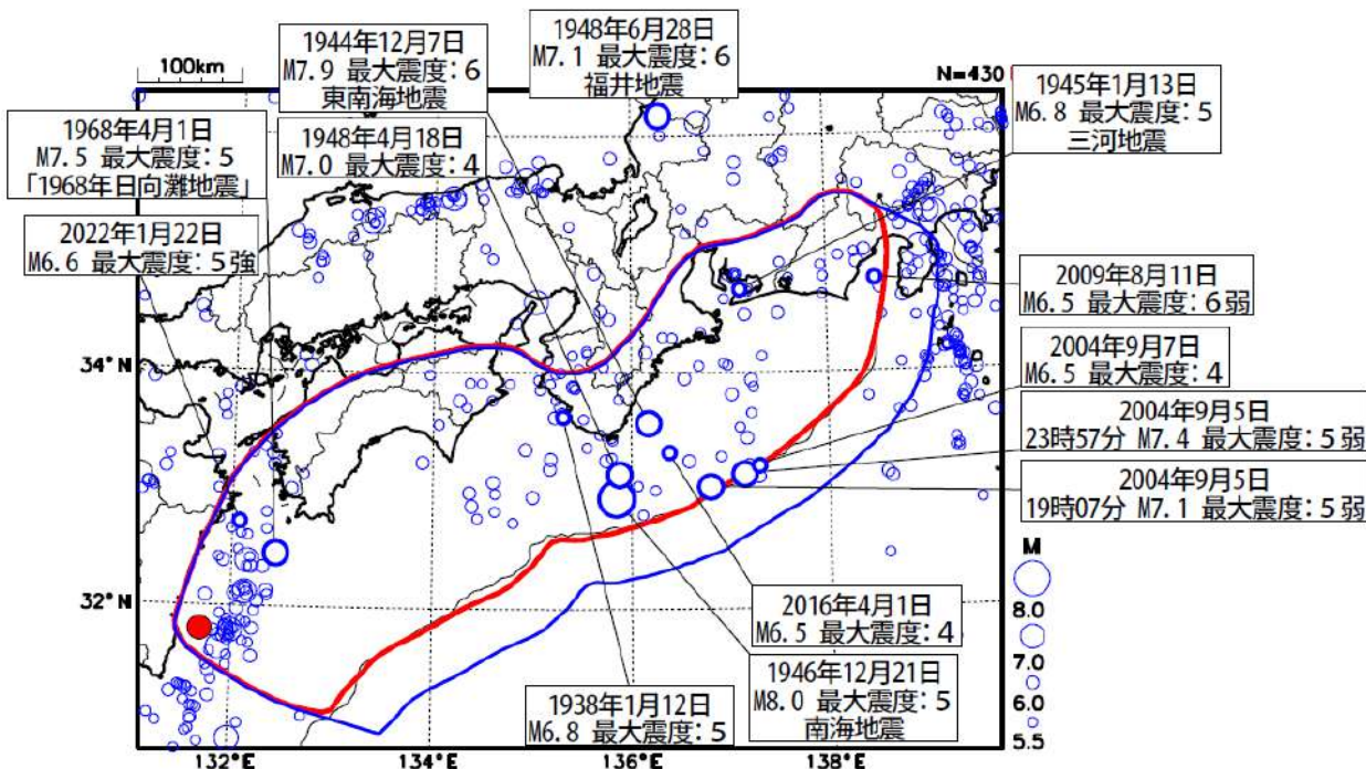
震央分布図
